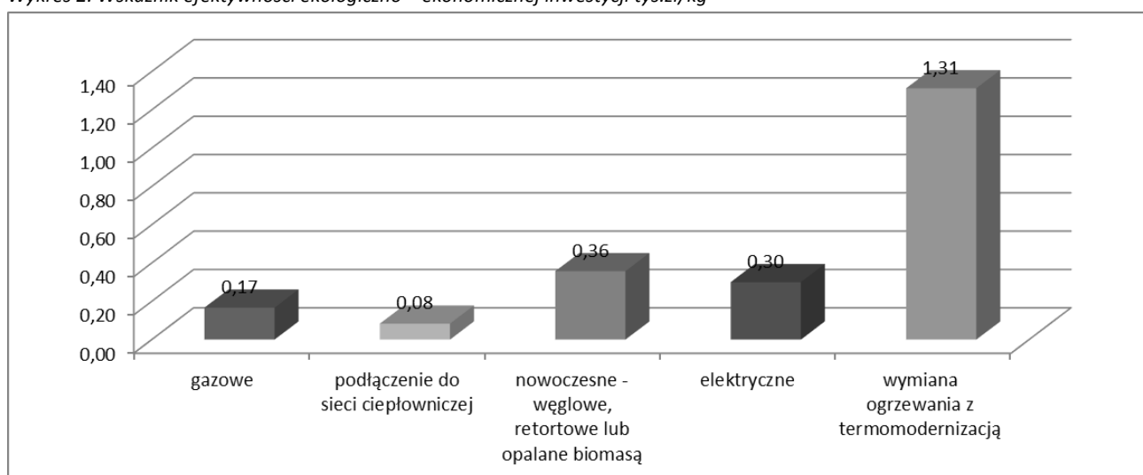
Wykres 2. Wskaźnik efektywności ekologiczno – ekonomicznej inwestycji tys. zł/kg
