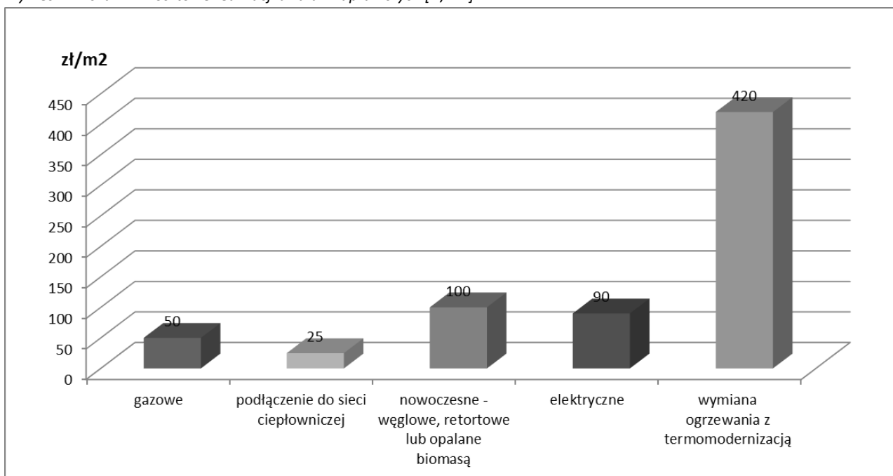
Wykres 1. Wskaźniki kosztowe realizacji działań naprawczych [zł/m 2 ]
