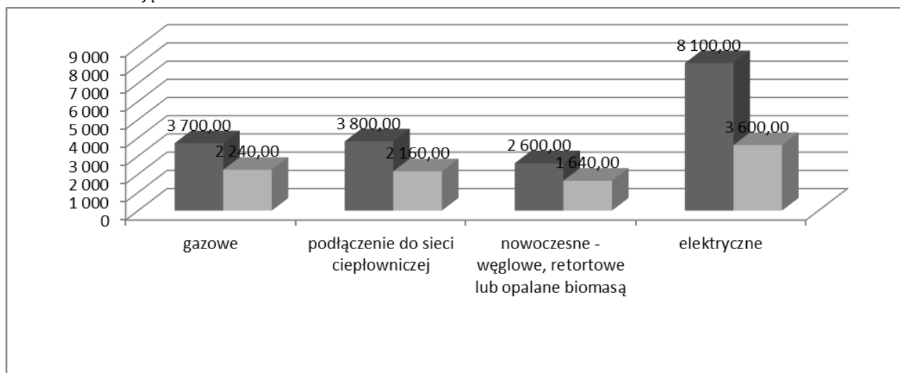
Wykres 3. Roczne koszty ogrzewania przykładowego domu jednorodzinnego o powierzchni 120 m 2 bez termomodernizacji i z termomodernizacją
